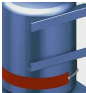
Vyhřívací páska na nádrži na chladivo: zvyšuje tlak a zajišťuje tak úplné naplnění i v případech, že je okolní teplota vysoká a motor horký
