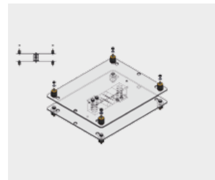
Bložisková vysokokapacitní váhící jednotka: určuje množství obnoveného chladiva s přesností na jeden gram a zajišťuje tak vysoce přesné plnění
