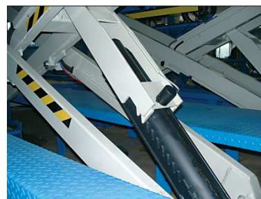
Zajištění polohy pomocí mechanických západek
