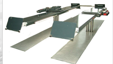
Masterlift 2.35 Combi Saav 135 VAN VAS 5249
